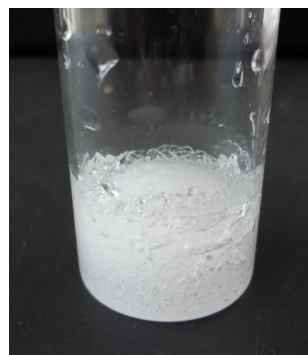
図「南極石」の結晶
